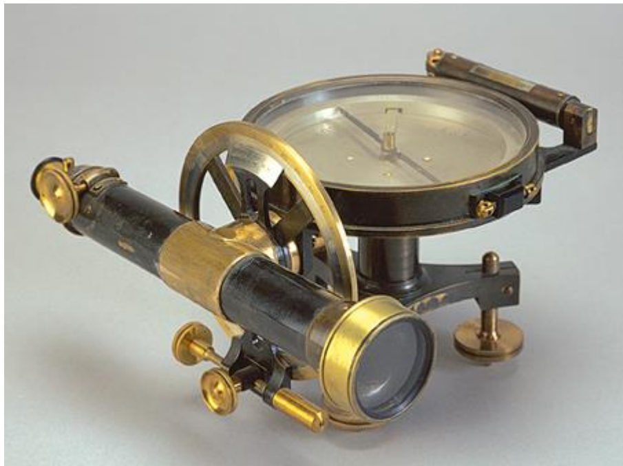
Brúixola taquimètrica, instrument topogràfic que aprofita el magnetisme terrestre per a mesurar angles
